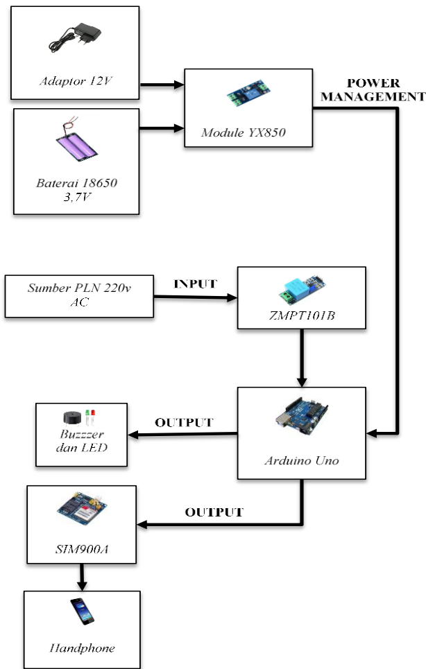
Gambar 2. Diagram blok alat pendeteksi status listrik
