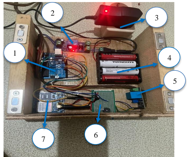
Gambar 4. Hasil perancangan perangkat keras alat pendeteksi status listrik berbasis SMS
